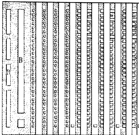
Fig. 25. — Coupe horizontale par mn et par op .
